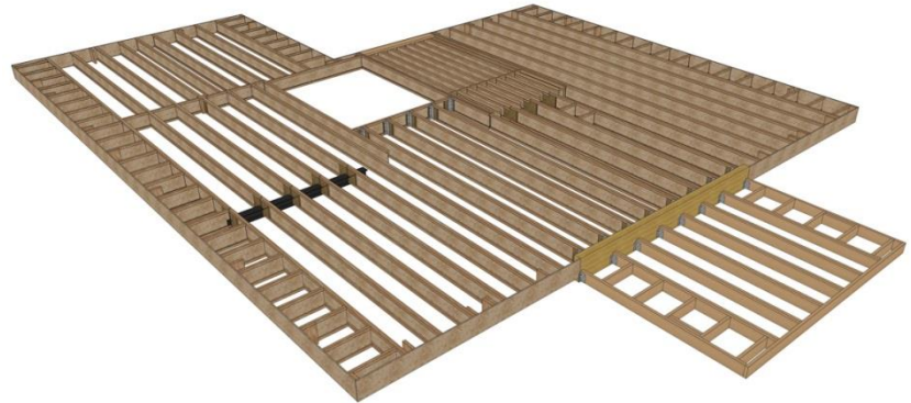
Illustrasjon av trebjelkelag: Ref. NDLA
